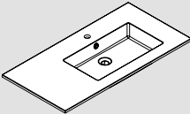
100 x 50 cm · 16,6h - Der · Right · Droite
