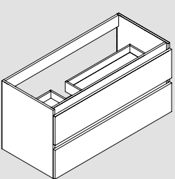
110 x 50 cm · 55h - Izq / Left / Gauche
